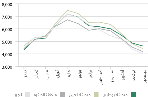
الشكل 6.2.5. متوسط المجموع اليومي لشدة الإشعاع الشمسي حسب المنطقة والشهر، 2016
